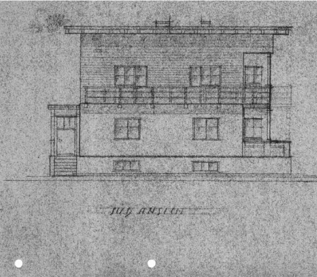
Süd Ansicht
